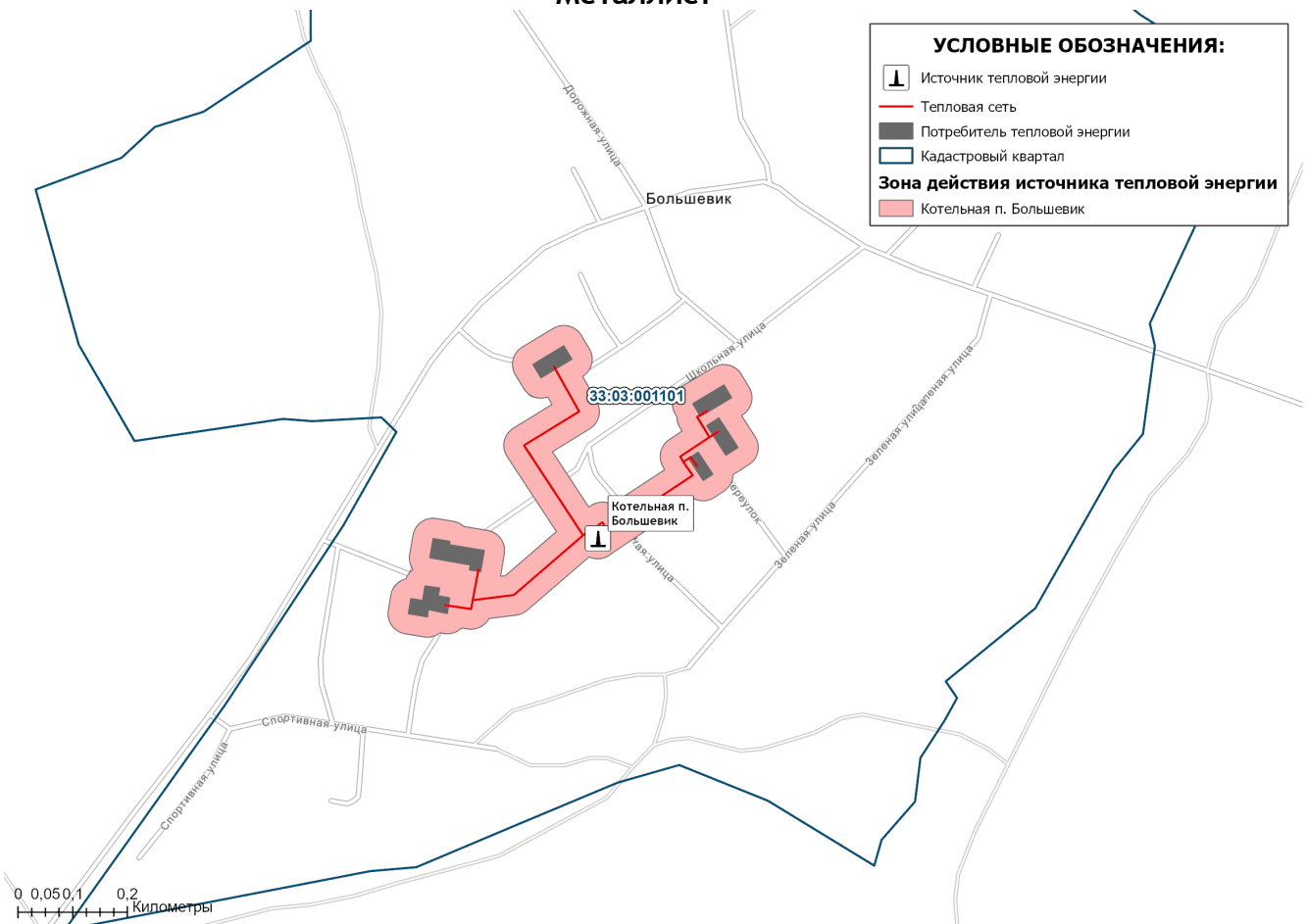
Рисунок 1.4.3 - Зона действия источника тепловой энергии на территории поселка Металлист
