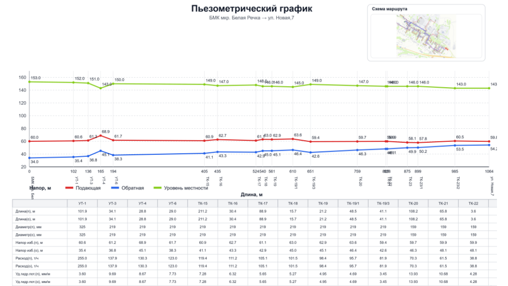
Рисунок 1.3.8.4 - Пьезометрический график
